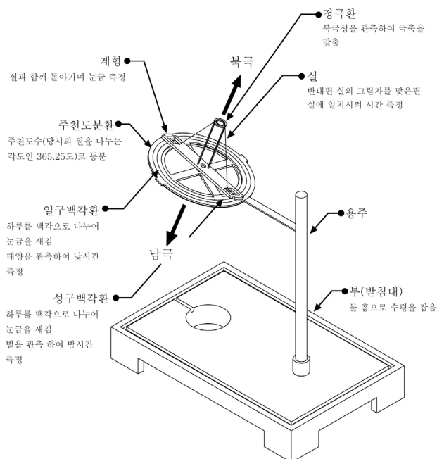
그림 3. 일성정시의(日星定時儀) 구조도와 복원 사진(세종대왕유적관리소).
