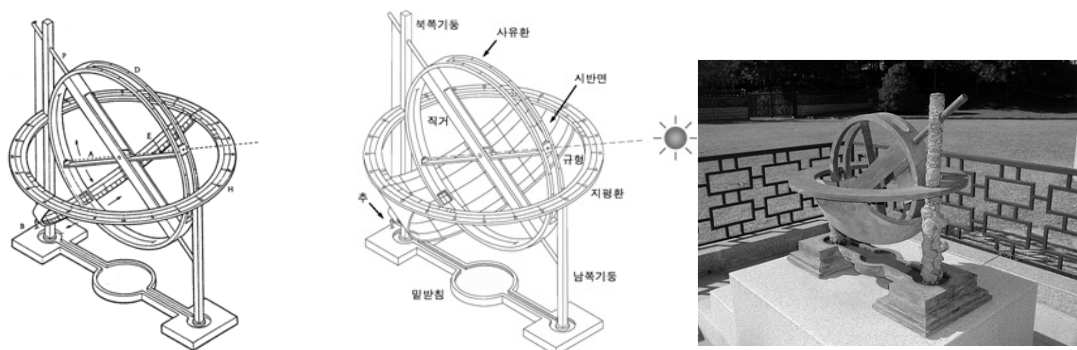
그림 7. Needam et al. (1986)의 모델(좌)과 본 연구에서 설계한 정남일구와 복원모델(우).
