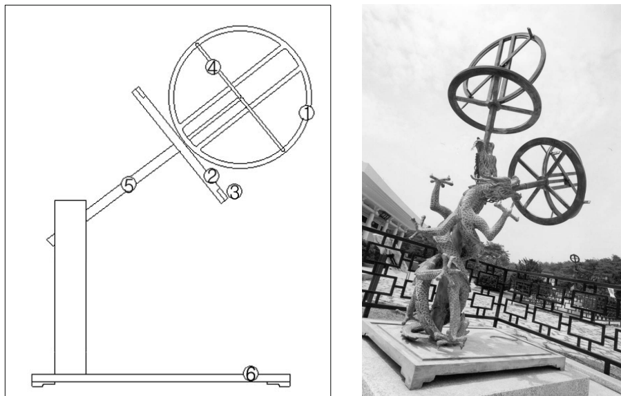
그림 2. 小簡儀의 각 部品별 名稱과 小簡儀의 復元(세종대왕유적관리소).
