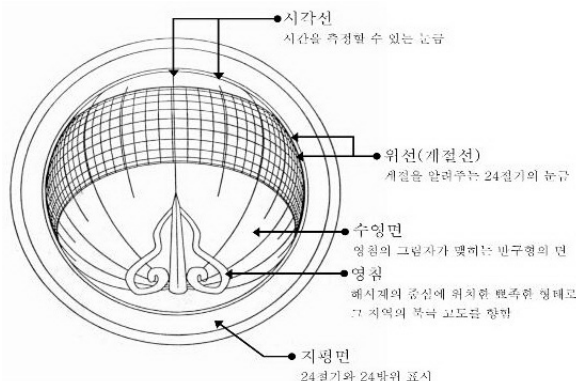
그림 4. 양부일구의 구조와 평면도 및 복원한 양부일구(한국천문연구원).
