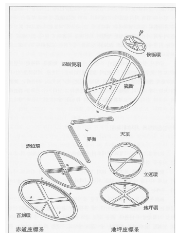
그림 1. 한국천문연구원에 복원한 간의(簡儀)와 간의의 부품도.
