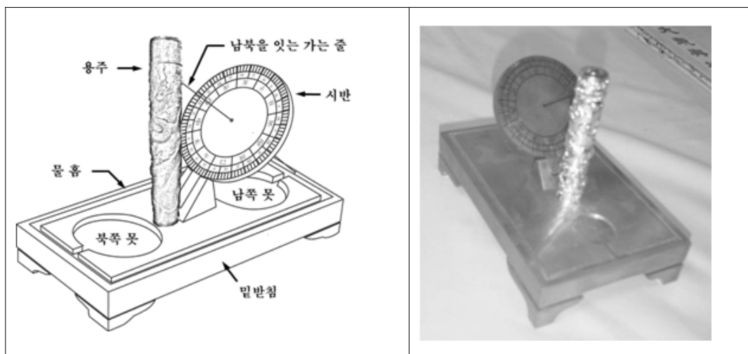
그림 6. 천평일구 구조도와 복원사진.
