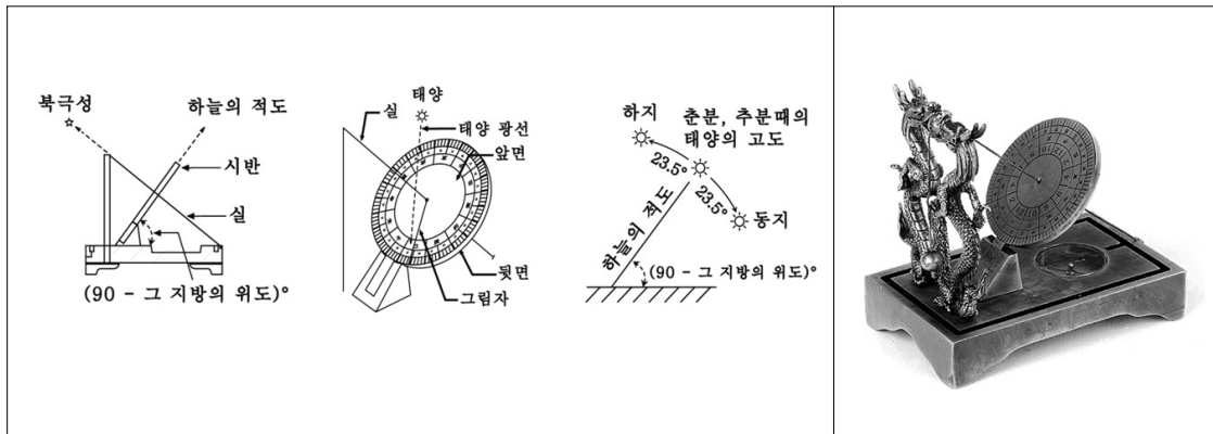
그림 5. 적도식 해시계 구조와 태양의 고도변화 및 복원한 현주일구.
